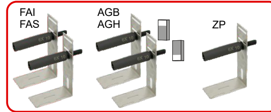
||||| QJ4.CTKIMP.H5 / QJ4.CTKIMP.H4 (ohne AGH) Positionsschalter als Magnet + Türzone/Nachregulierung i + Vorendschaltern Unten/Oben als Magnet und reset magnete
