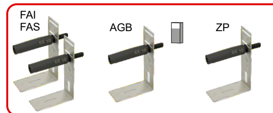
QJ4.CTKIMP.H4 Sistema di conteggio con lettori magnetici + zona porte / rilivellamento + impulsore di prossimità per reset basso e magneti
